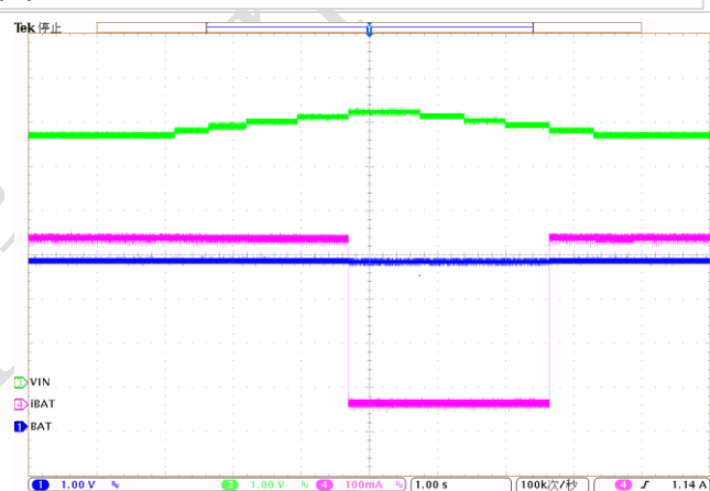
VIN OVP 保护波形
