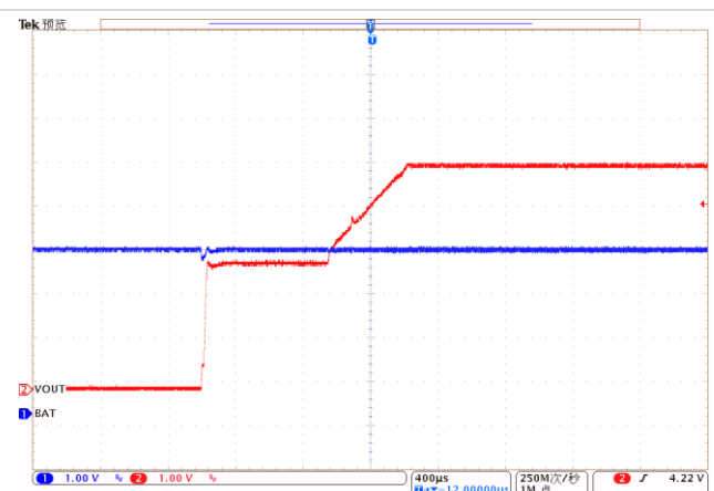
VOUT 带 100mA 负载, 软启动波形
